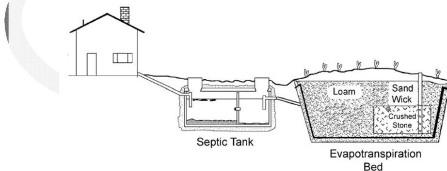
Evapotranspiration (ET) bed
